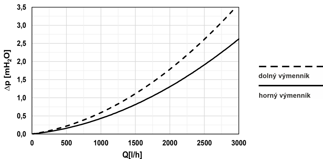
Graf poklesu tlaku
