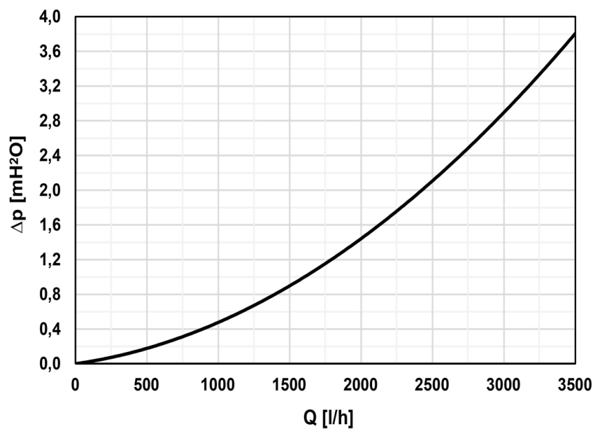
Graf poklesu tlaku
