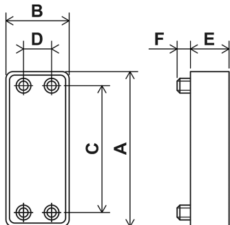
Rozmerová schéma
