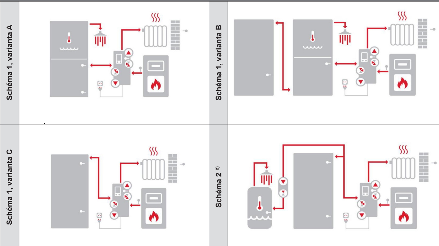
Možnosti základného zapojenia 1)
