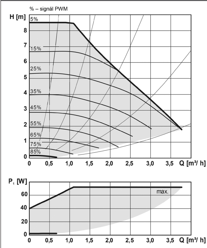
Výkonové krivky čerpadiel Wilo Para 25/8 iPWM1
