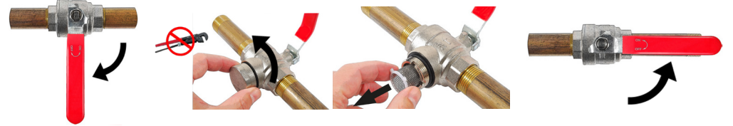
Obr. 6 - uzavření kohoutu
