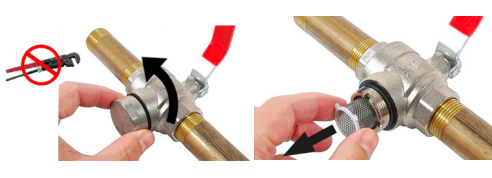
Fig. 7 - demontarea filtrului
