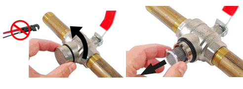
Abb. 7 - Entfernen des Filtersiebs
