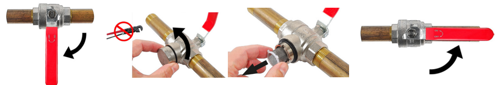
Obr. 6 - uzatvorenie ventilu
