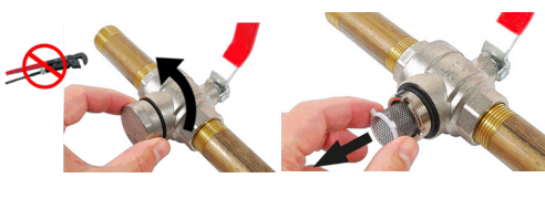
Obr. 7 - wyjęcie siatki filtra
