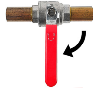
Abb. 6 - Hahn schließen
